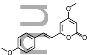
YANGONIN
