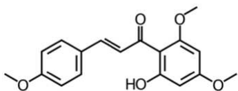
FLAVOKAWAIN A
